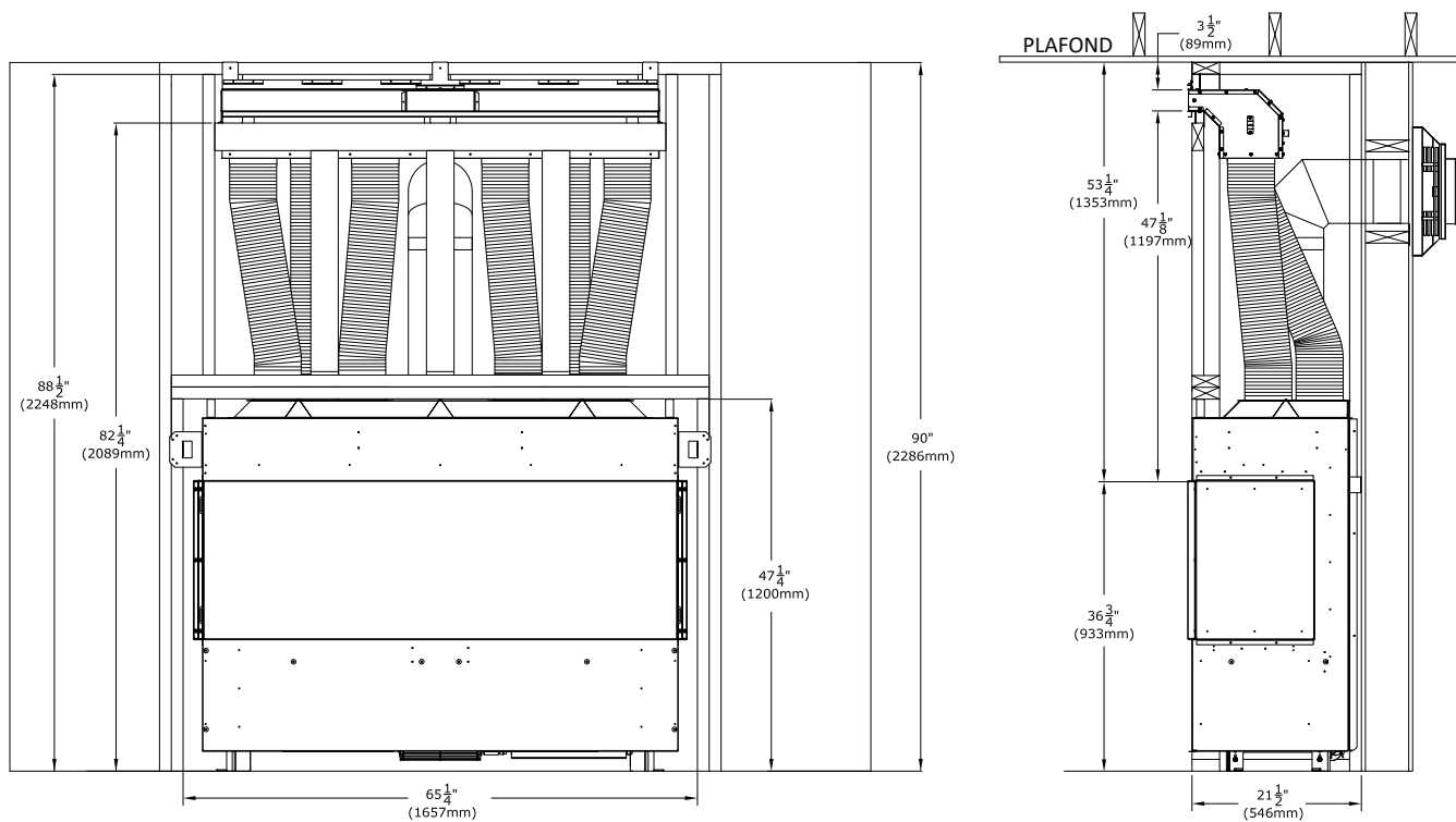
Figure 4.15 - Encadrement du plénum (enceinte de dimensions minimums)
