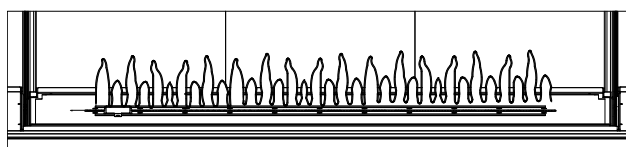
Flammes orange foncé à pointes noires (Venturi trop fermé - Ouvrir légèrement le venturi)
