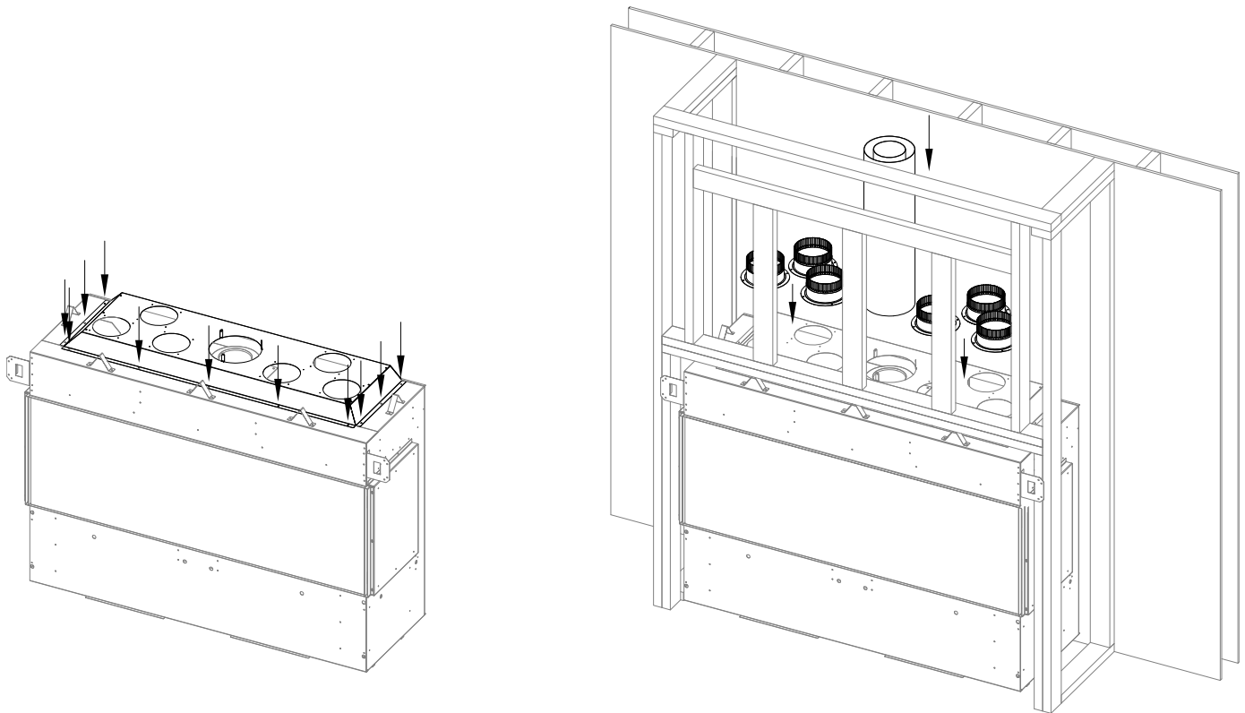
Figure 4.25 - Installation de la chute d'air et des collets du KZK
