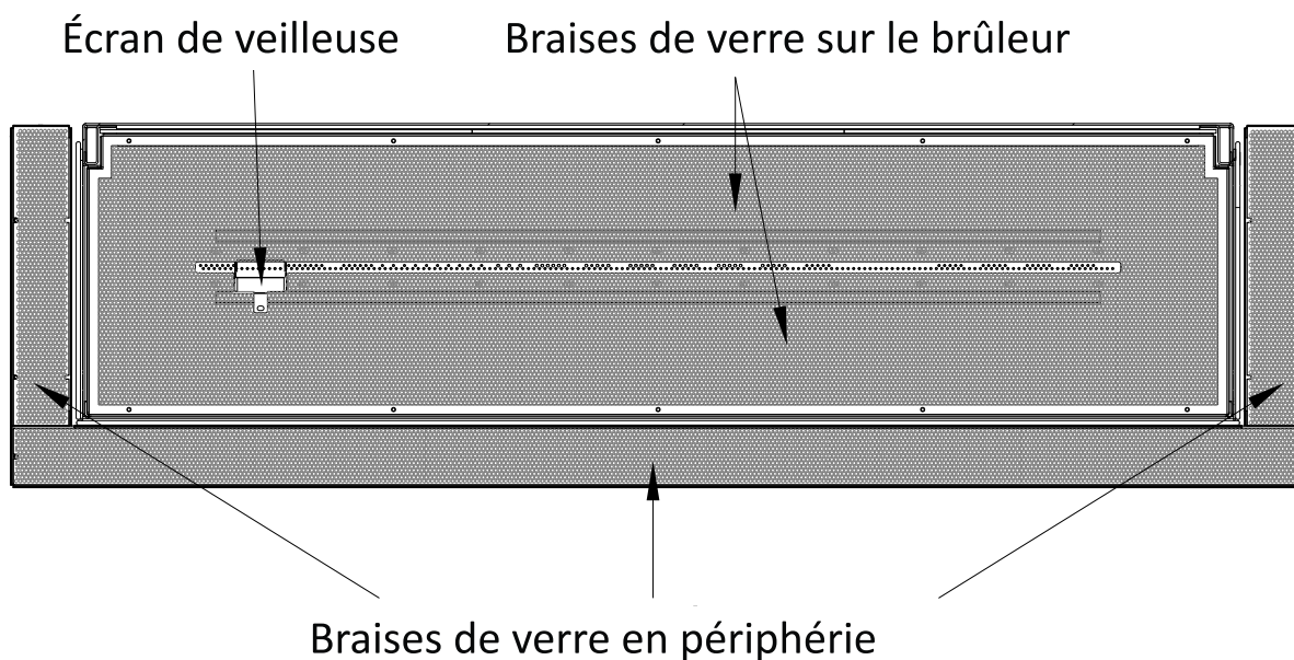
Figure 7.10 - Emplacement des braises de verre
