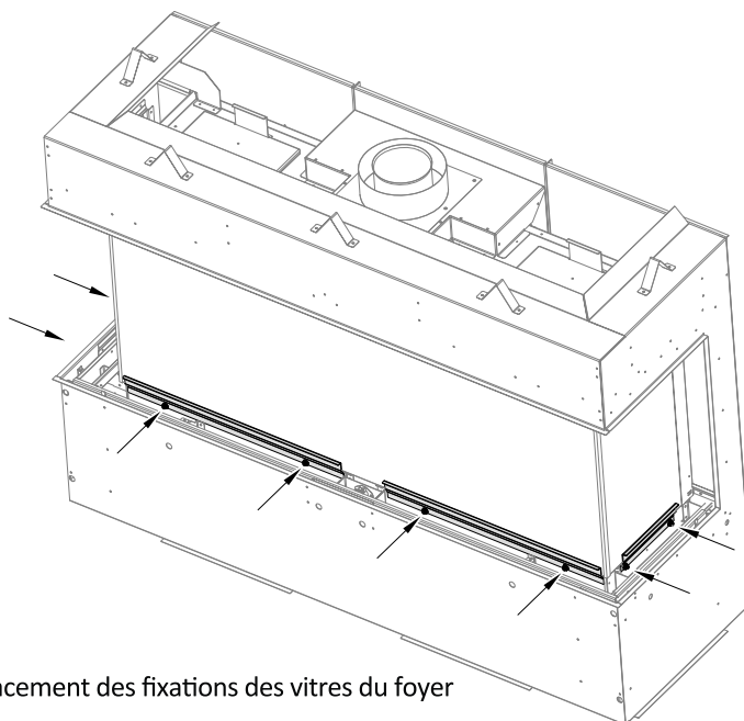
Fixations inférieures des vitres du foyer
