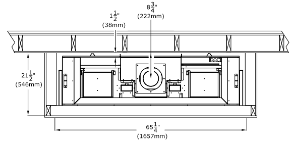
INSTALLATION TYPIQUE AVEC TERMINAISON VERTICALE
