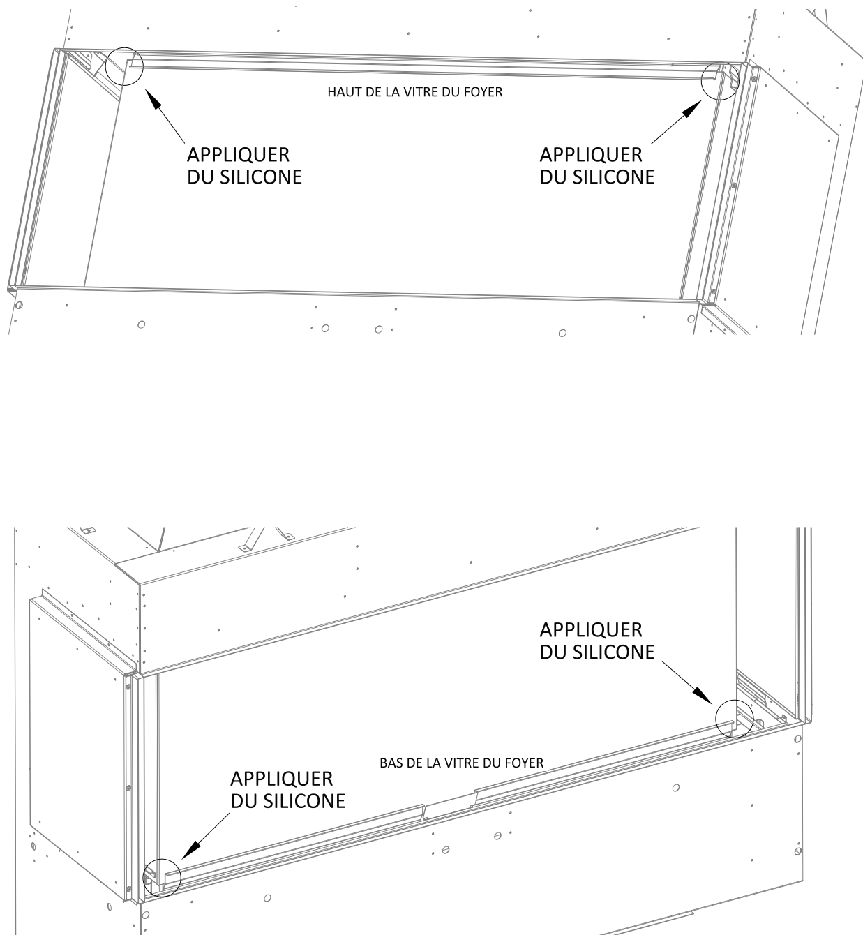
Figure 7.8 - Joints en silicone aux coins des vitres du foyer
