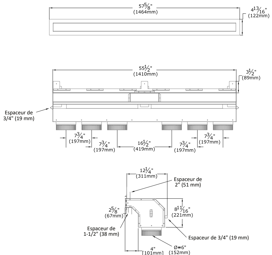
Figure 4.13 - Vue d'ensemble du KZK-056
