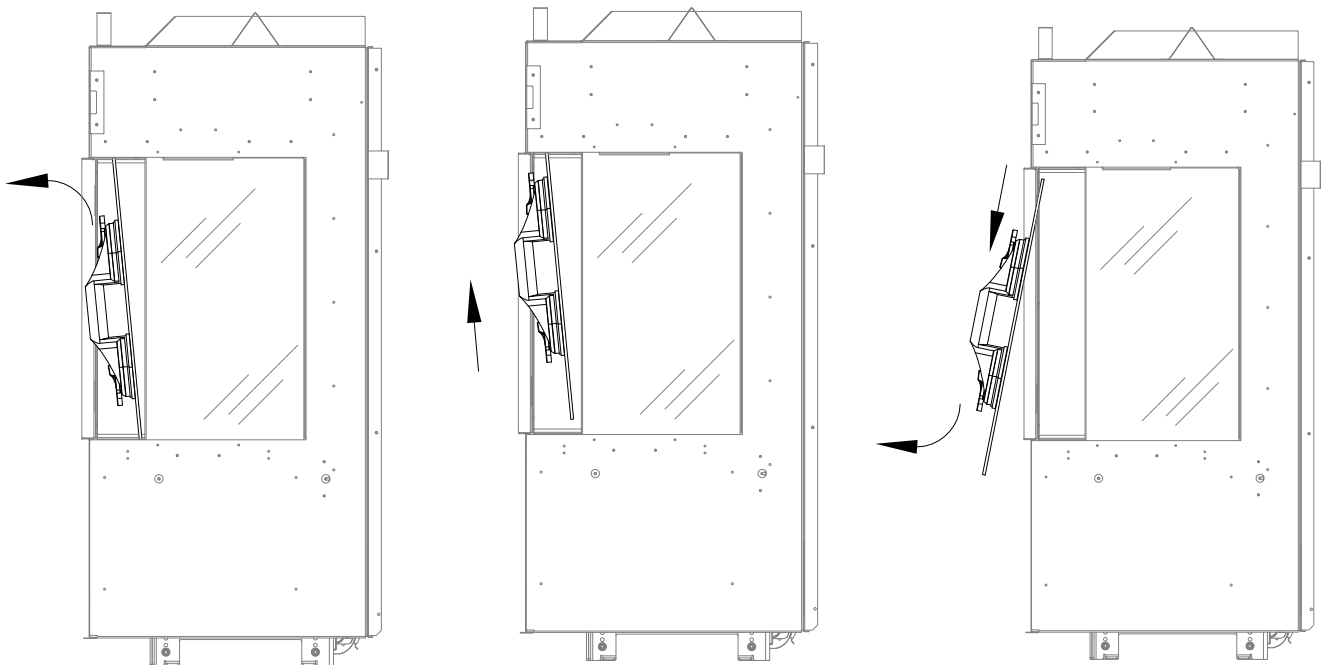
Figure 7.4 - Retrait de la vitre de façade du foyer
