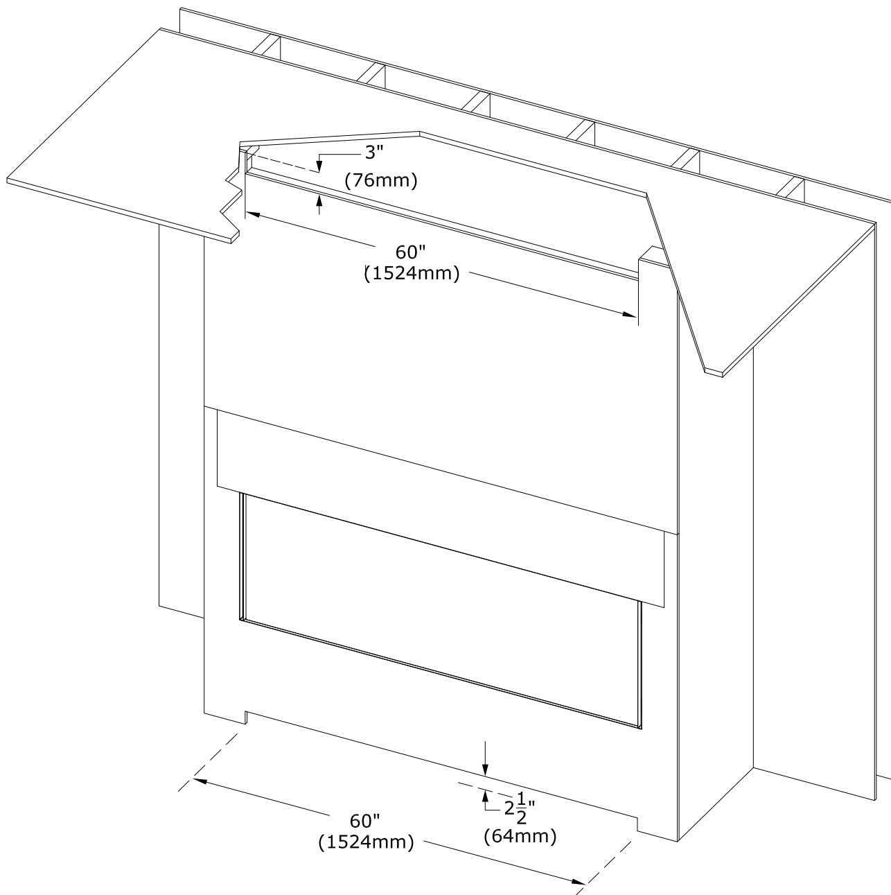
Figure 4.29 - Cavité ventilée - Sortie d'air à l'avant de l'enceinte
