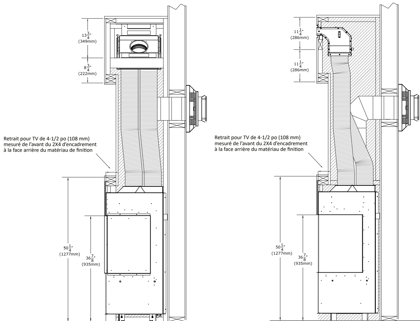
Installation du KZK latéral
