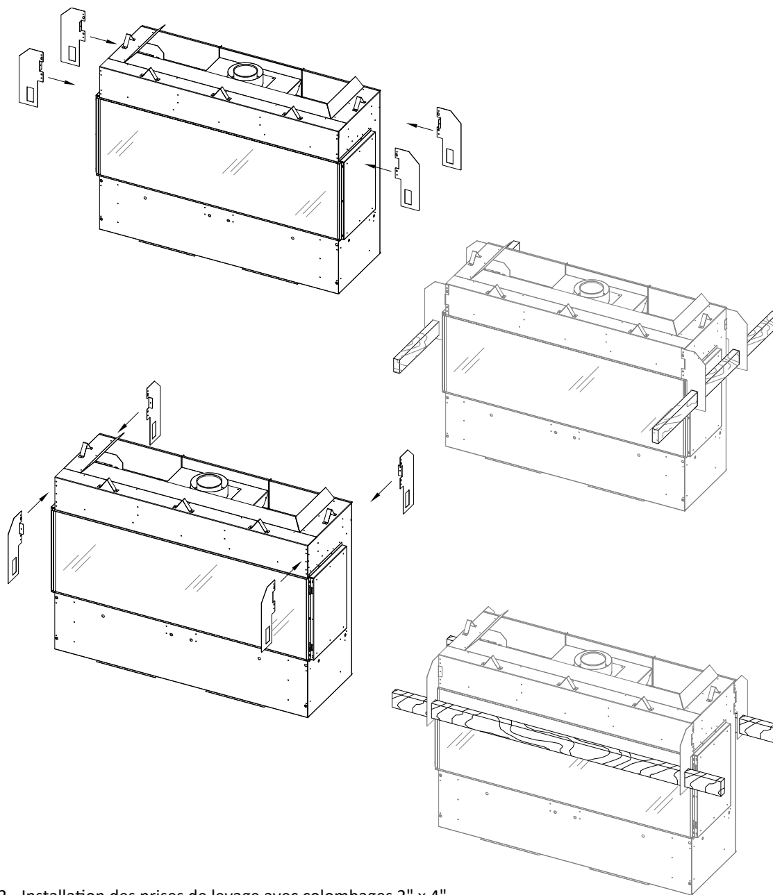
Figure 3.2 - Installation des prises de levage avec colombages 2" x 4"
