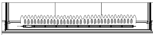
Flammes bleues et courtes (Venturi trop ouvert - Fermer légèrement le venturi)
