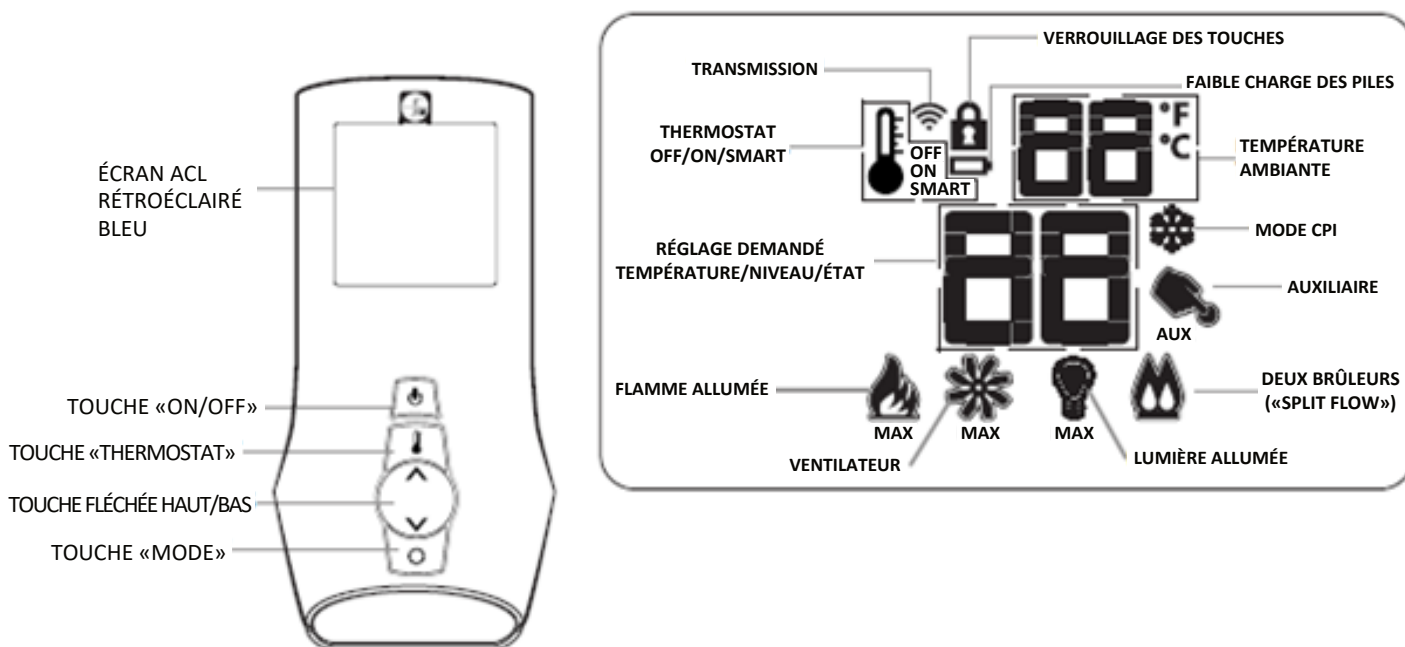
Figure 9.1 - Vue d'ensemble de la télécommande
