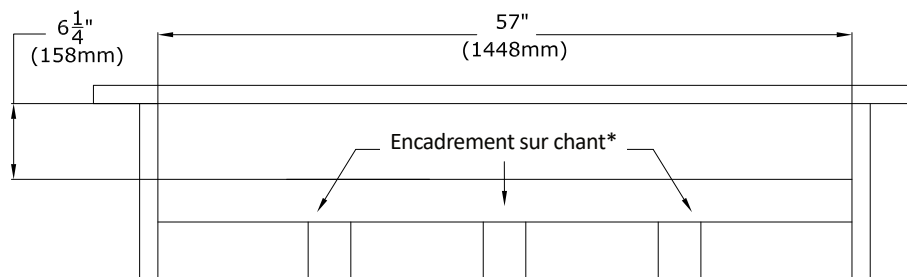
Figure 4.14 - KZK de façade - Ouverture encadrée du plénum
