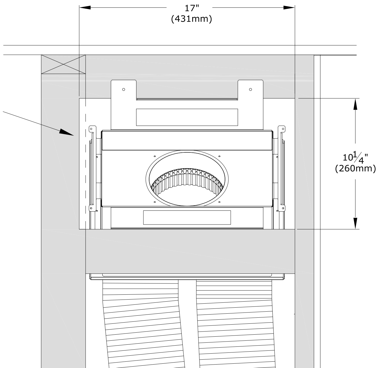
Figure 4.20 - KZK latéral - Encadrement de l'ouverture des plenums
