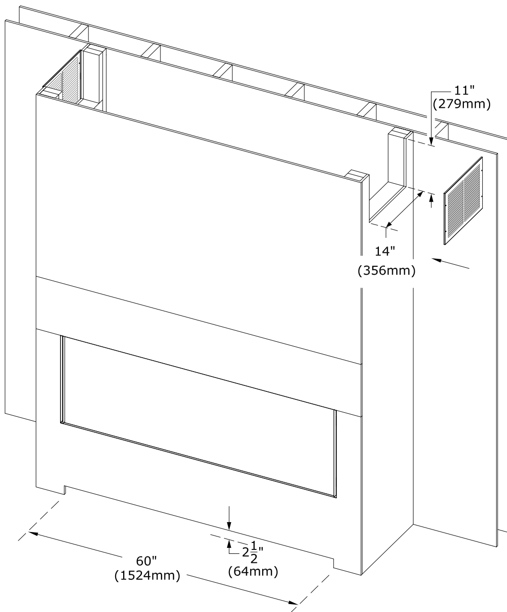
Figure 4.32 - Sorties d'air chaud par les ouvertures latérales
