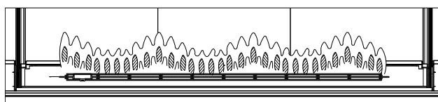
Flammes sautillantes («ghosting») (Venturi trop fermé - Ouvrir légèrement le venturi) OU (Pression de gaz trop élevée - Vérifier la pression au manomètre)
