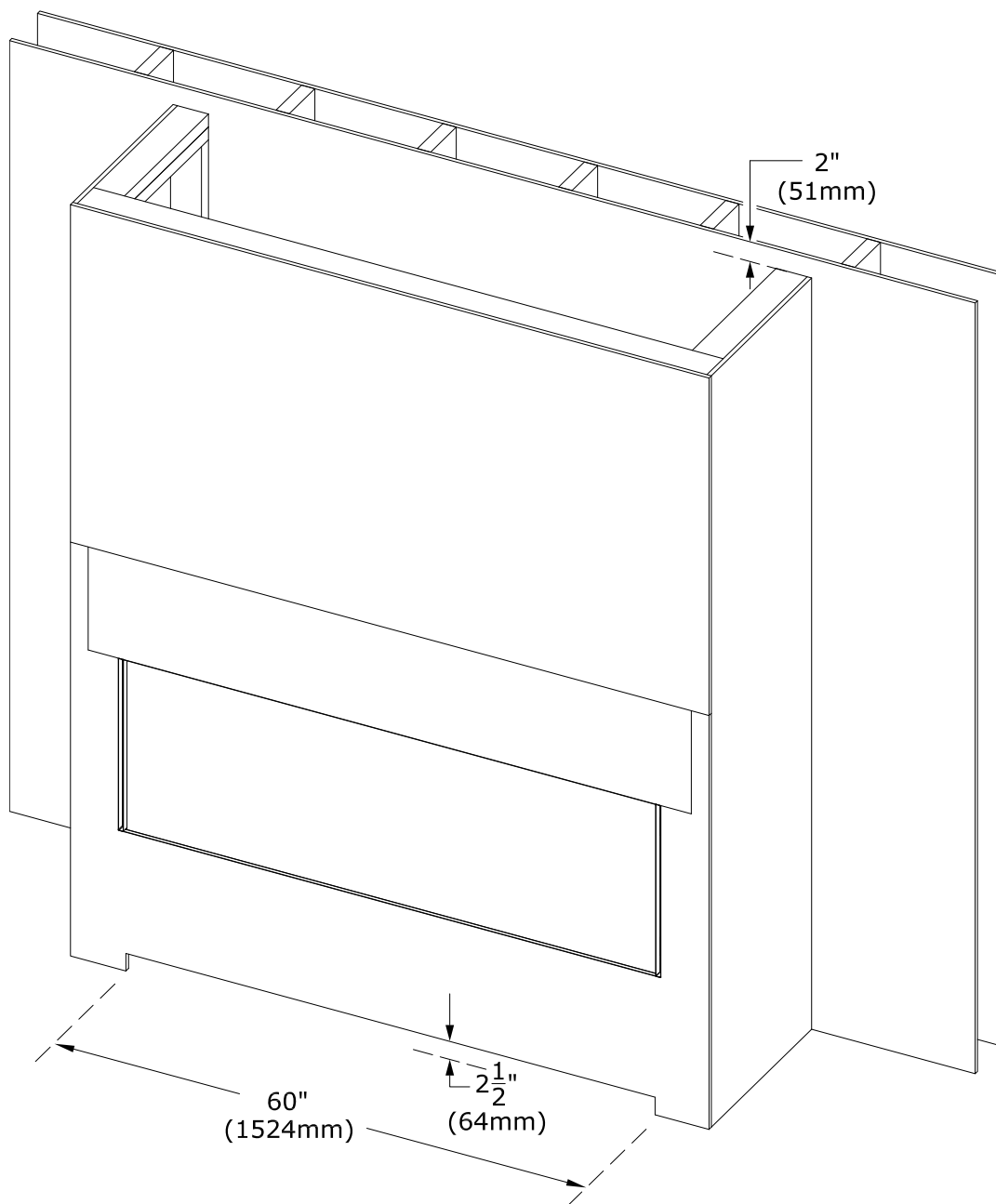
Figure 4.26 - Cavité ventilée - Sortie d'air aux 3 côtés de l'enceinte
