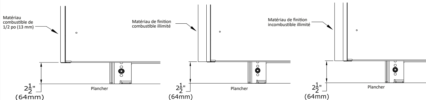
Figure 4.17 - Ouverture de prise d'air avec KZK (Options de finition)
