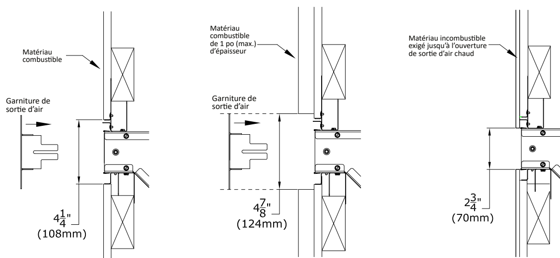
Figure 4.16 - Ouverture du plénum du KZK (Options de finition)
