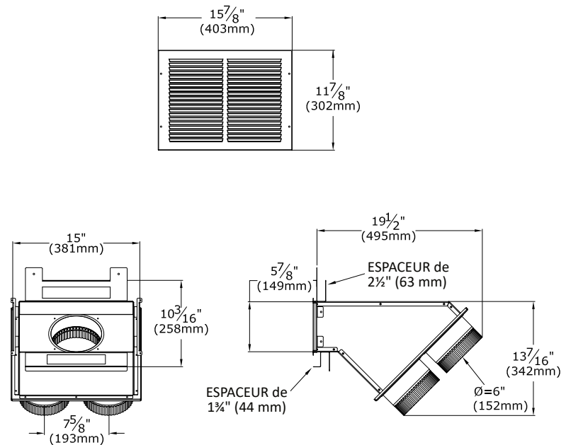
Figure 4.19 - Vue d'ensemble du kit KZK-1510
