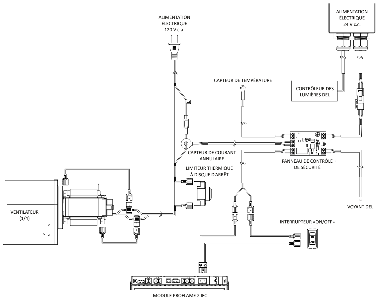
Figure 8.2 - Vue d'ensemble du système de contrôle de sécurité
