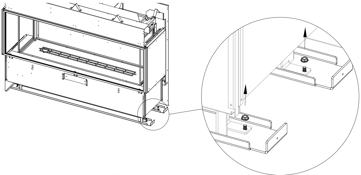
Figure 1.2 - Retrait des supports d'expédition
