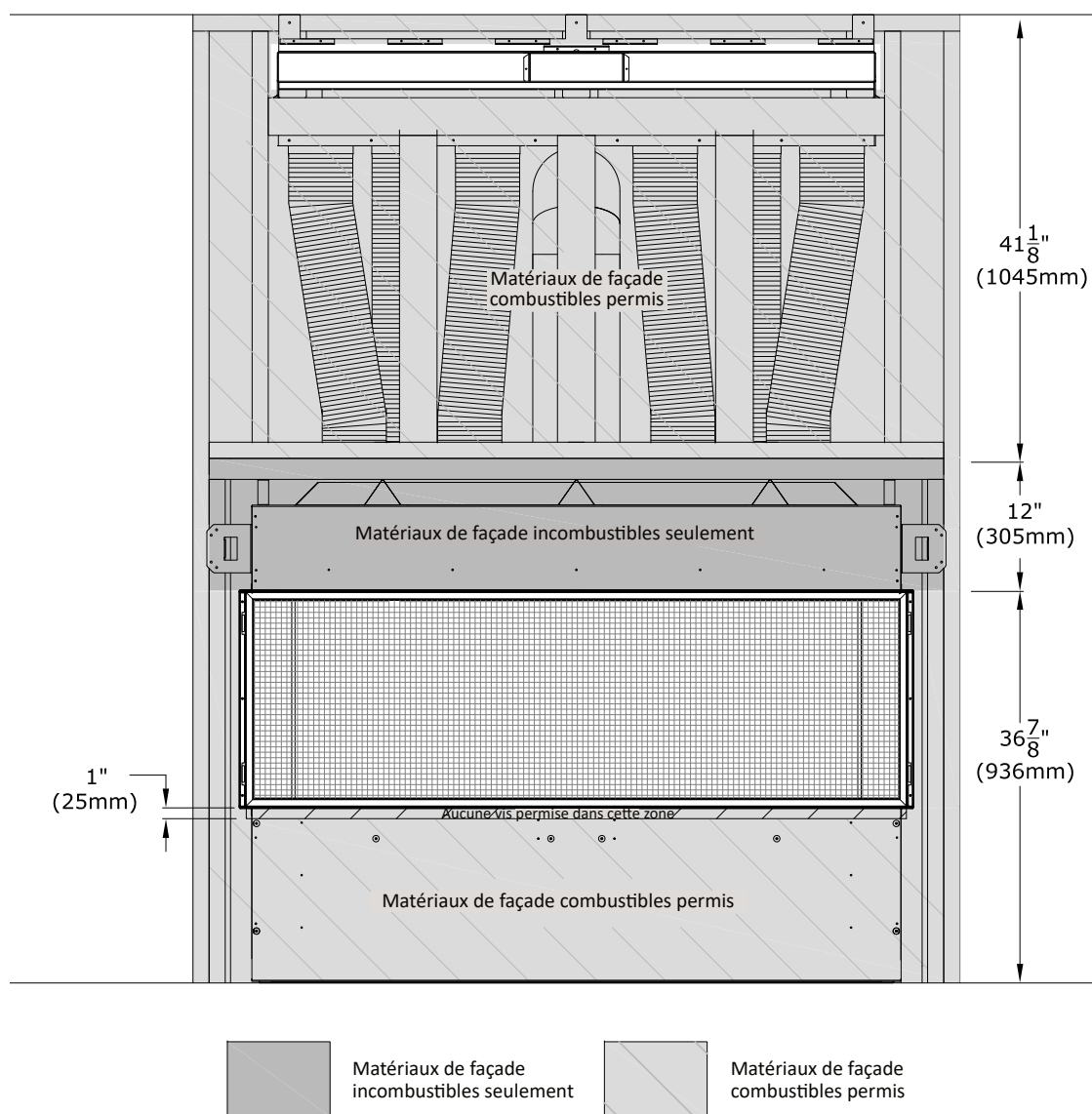
Figure 4.6 - Exigences d'installation des matériaux de façade
