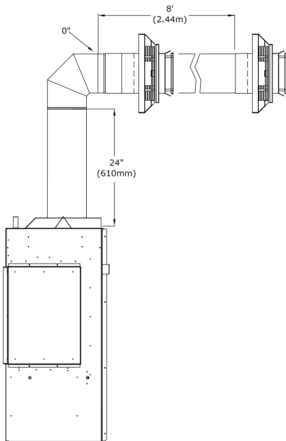
Figure 6.7 - Terminaisons horizontales
