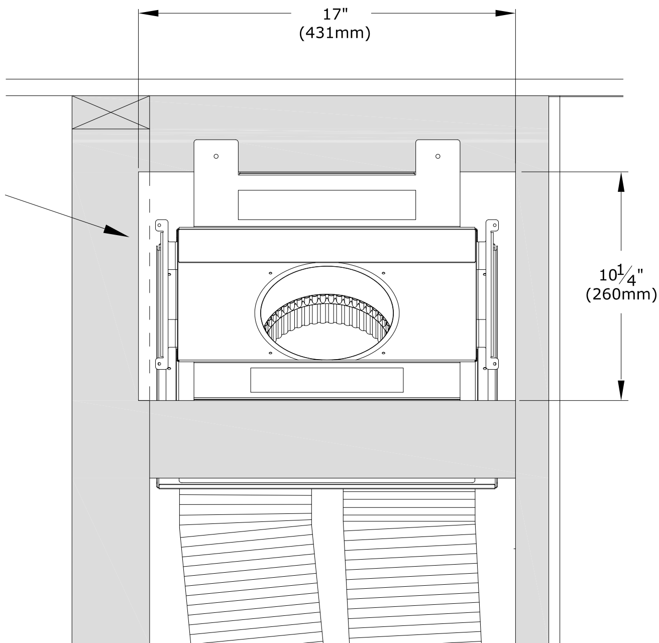
Figure 4.16 - KZK latéral - Encadrement de l'ouverture des plenums
