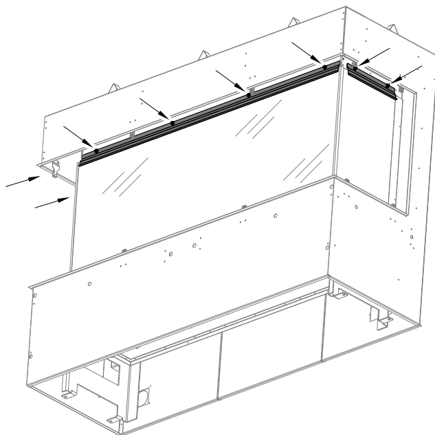
Fixations supérieures des vitres du foyer
