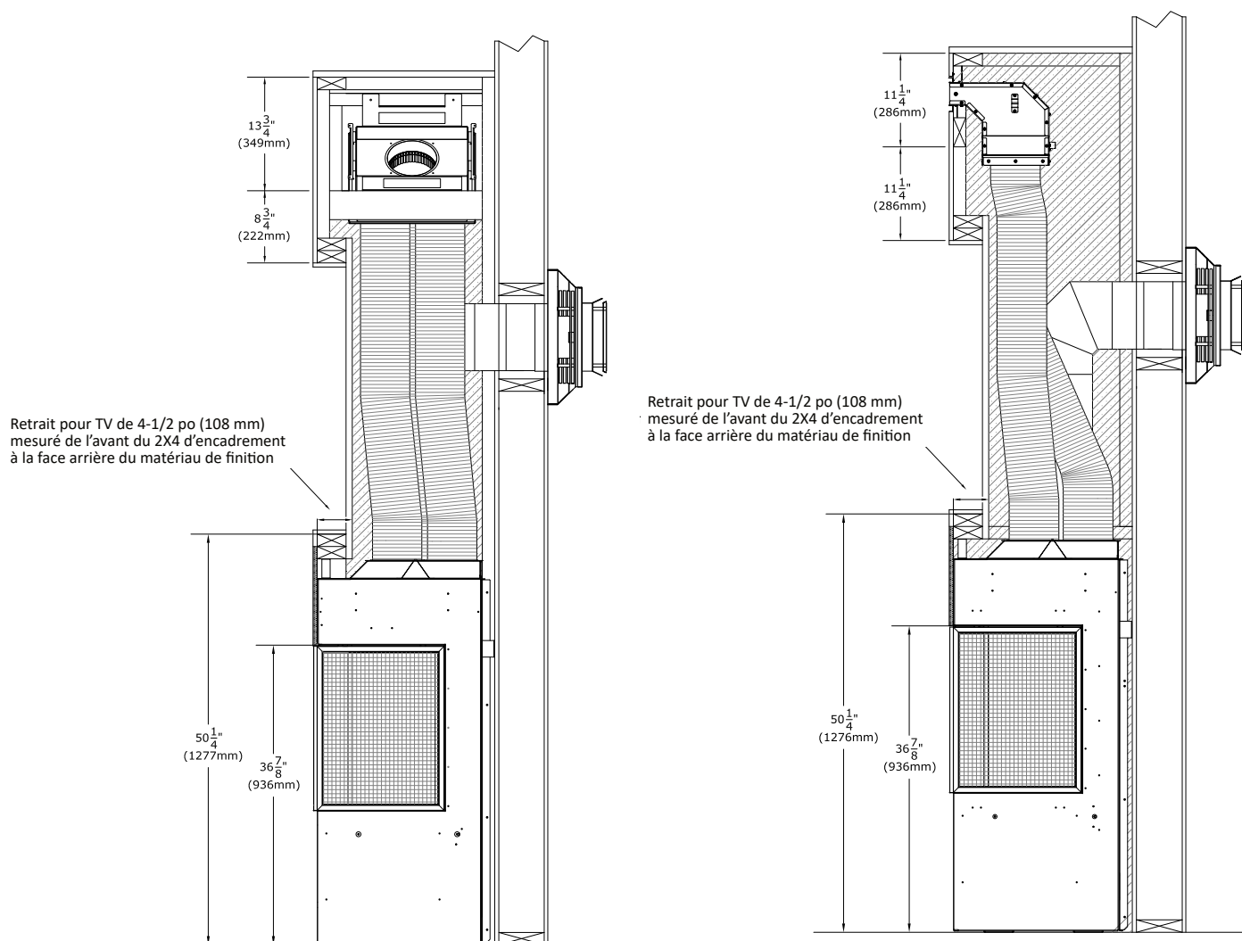
Figure 4.3 - Installation d'une télévision en retrait
