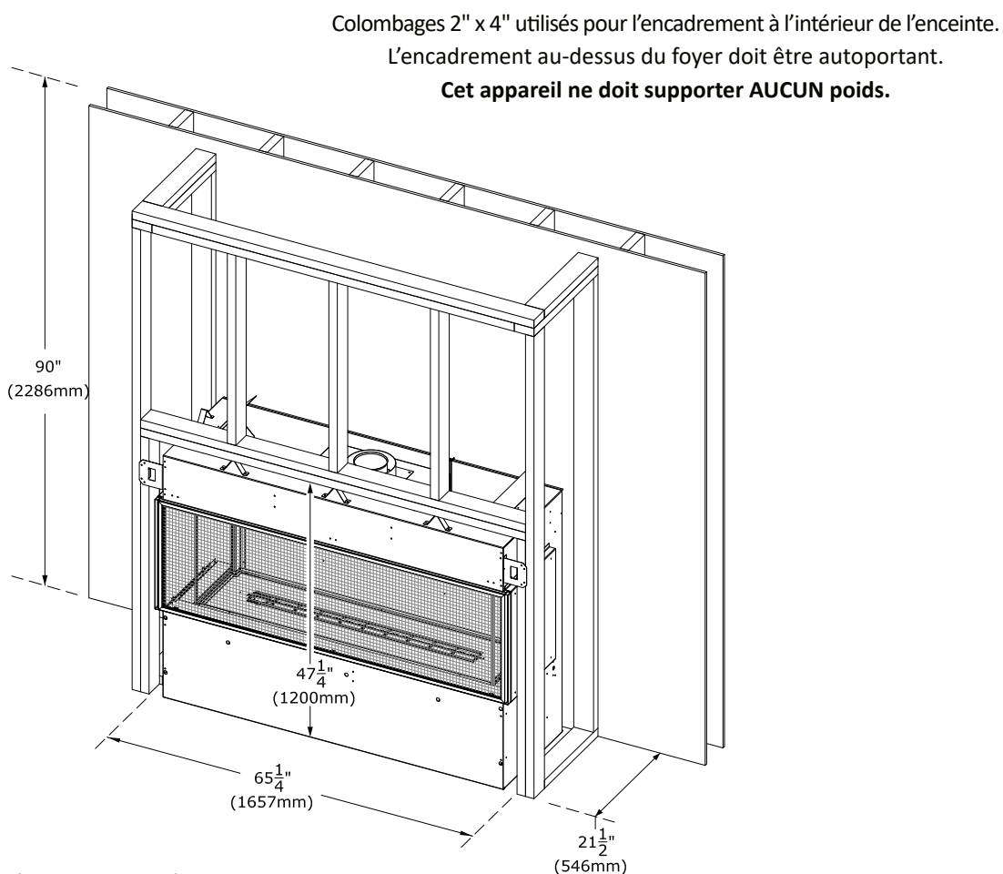
Figure 4.1 - Exigences d'installation de l'encadrement
