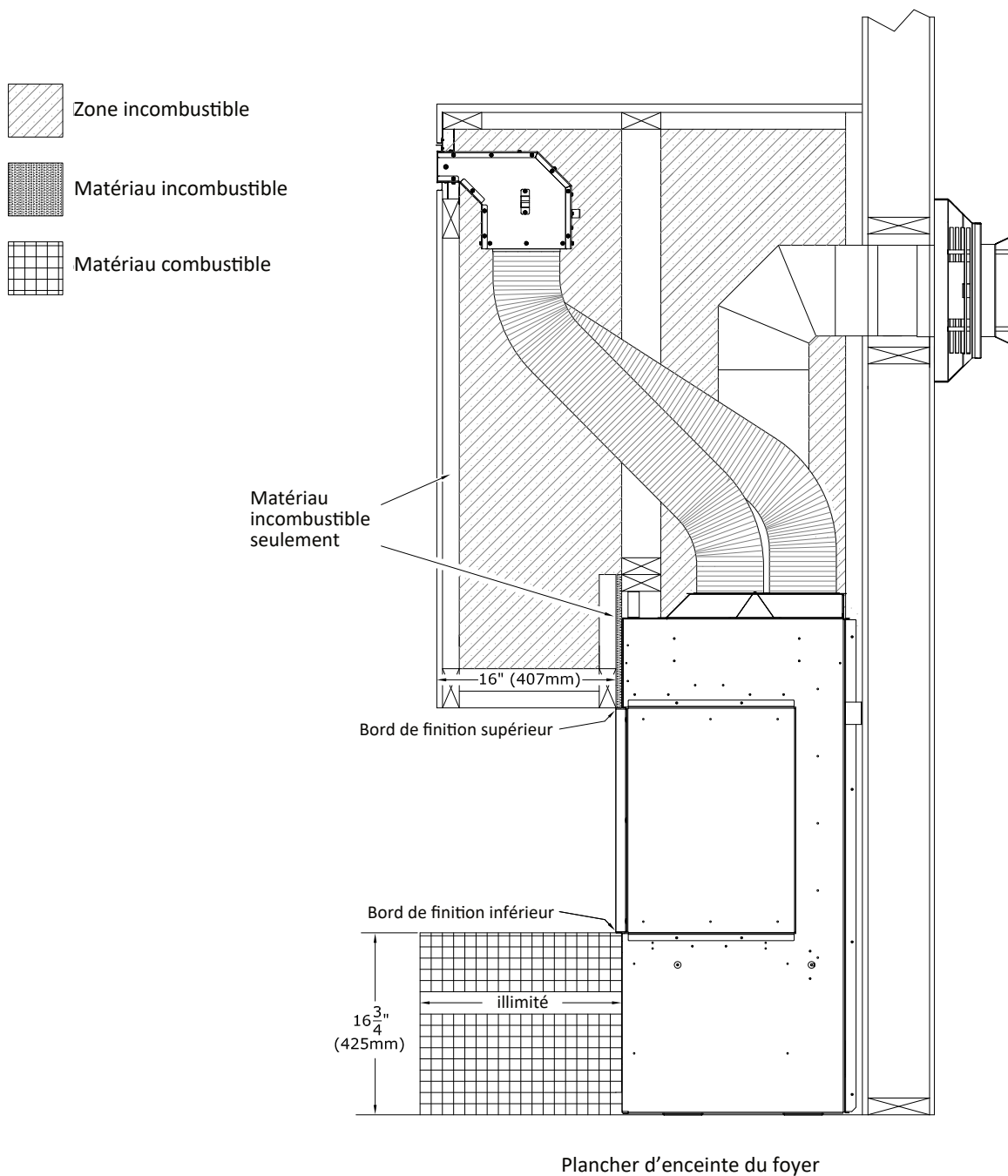
Figure 4.28 - Projections de l'enceinte et de l'extension d'âtre
