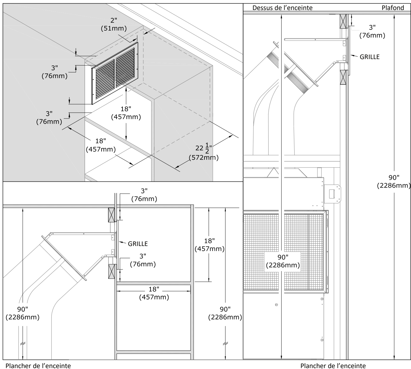
Figure 4.36 - Dégagement au mur latéral adjacent
