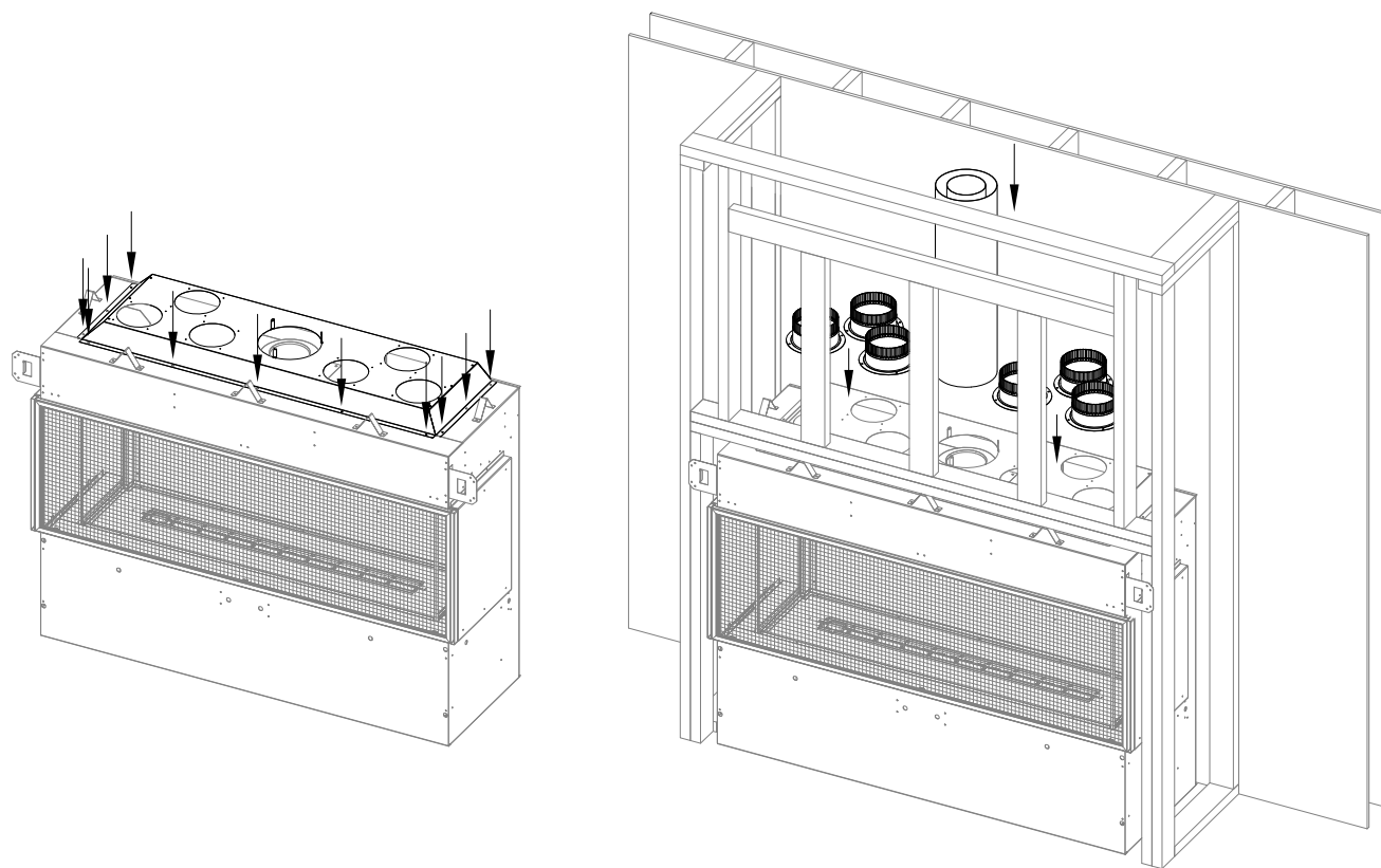
Figure 4.19 - Installation de la chute d'air et des collets du KZK
