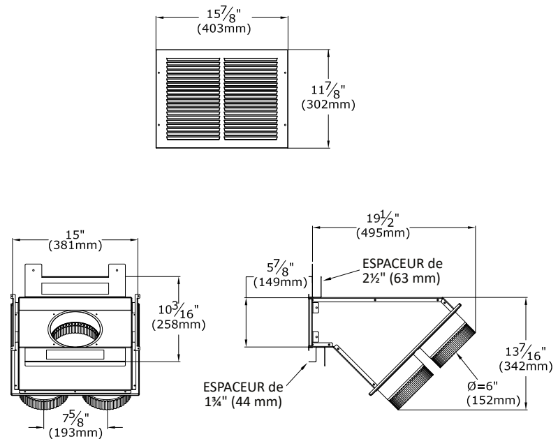
Figure 4.15 - Vue d'ensemble du kit KZK-1510
