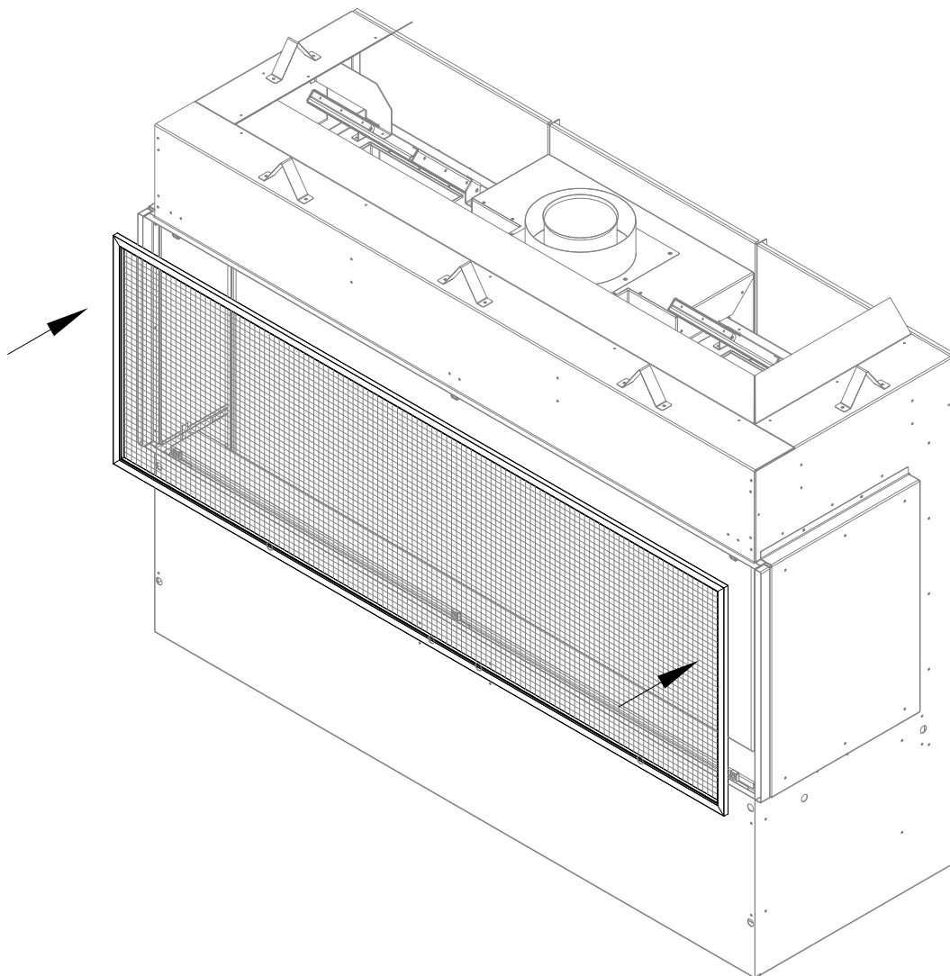
Figure 7.2 - Installation de l'écran pare-étincelles
