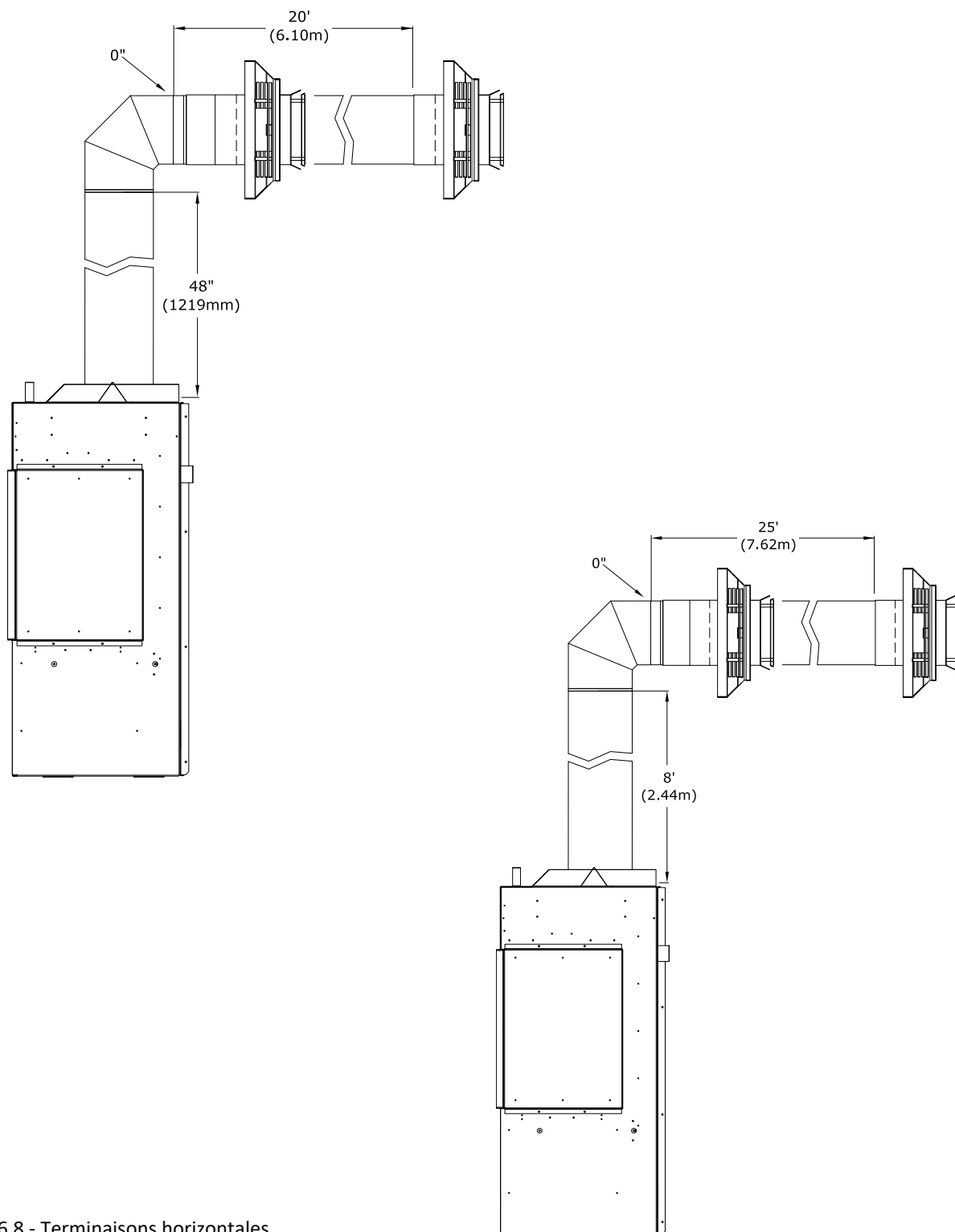
Figure 6.8 - Terminaisons horizontales
