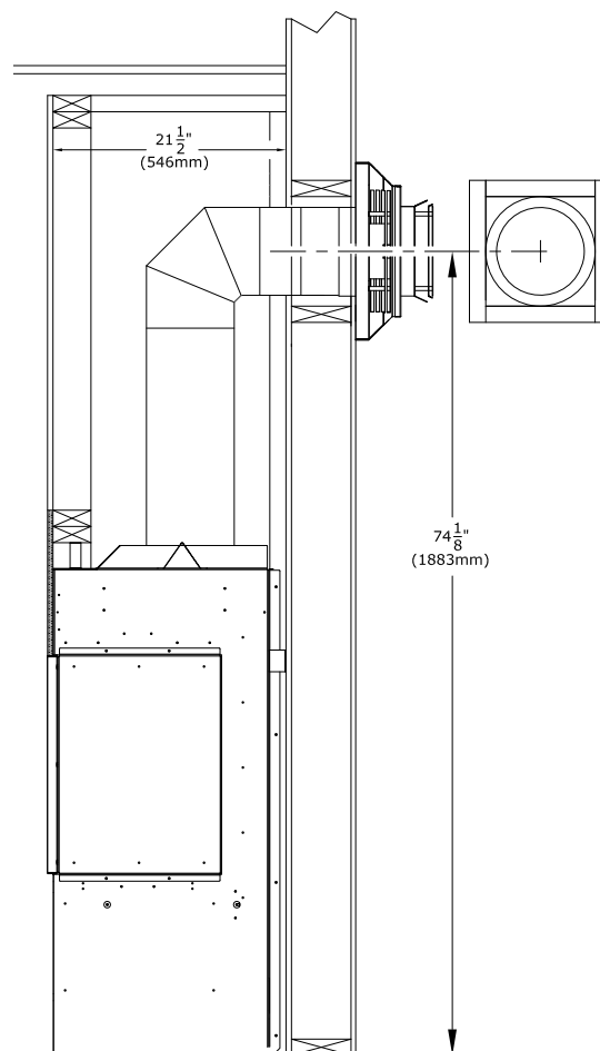
Figure 4.5 - Encadrement minimum du coupe-feu WPT
