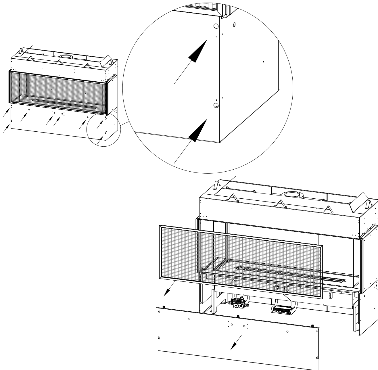
Figure 3.6 - Panneau d'accès à l'avant
