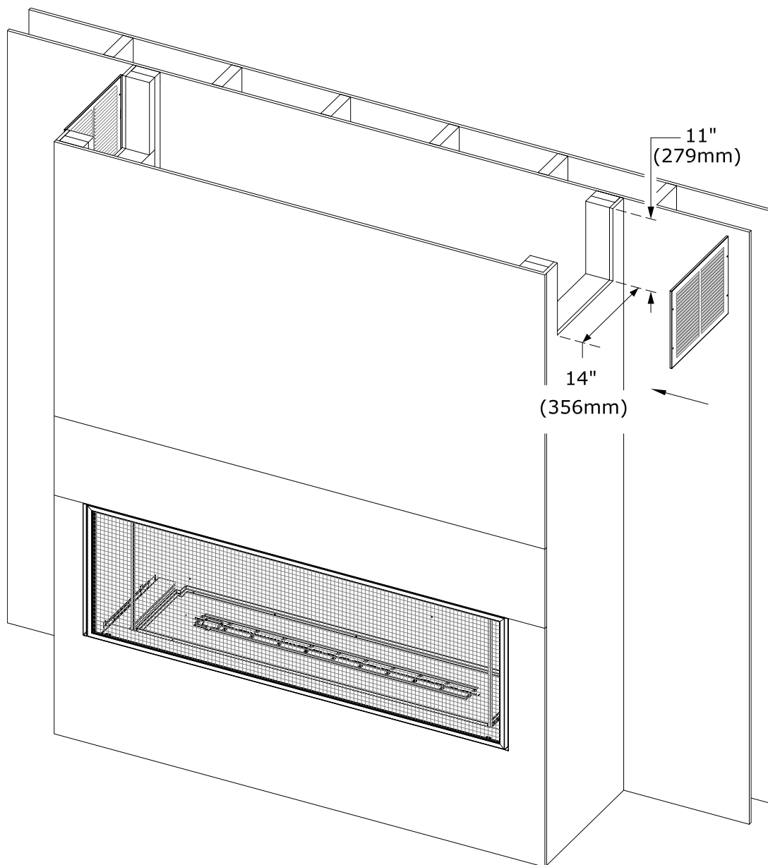
Figure 4.26 - Sortie d'air chaud par les ouvertures latérales
