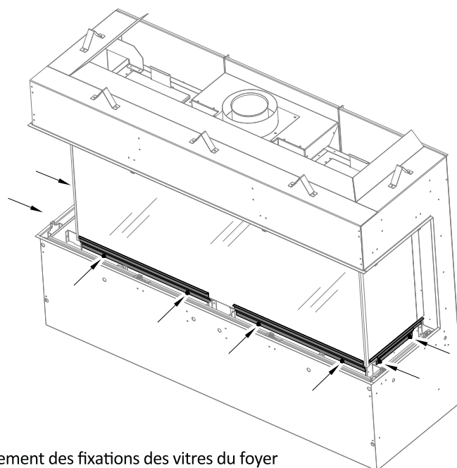
Fixations inférieures des vitres du foyer
