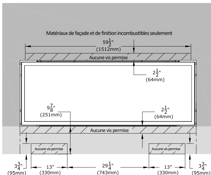
Figure 5.6 - Exigences des matériaux de façade et de finition incombustibles
