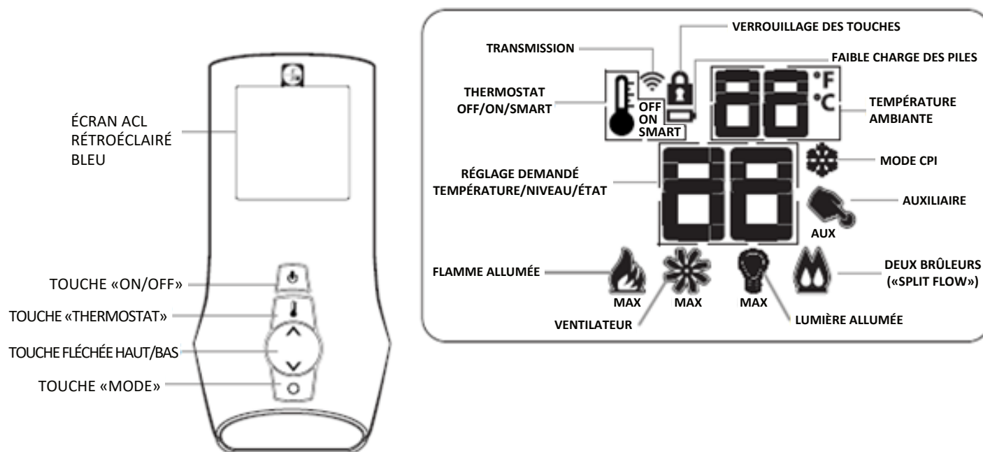
Figure 10.1 - Vue d'ensemble de la télécommande
