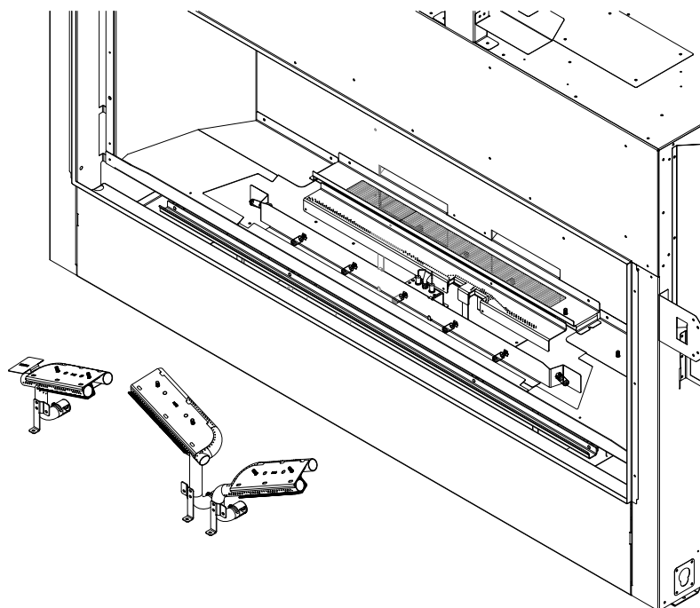
Figure 8.4 - Retrait des brûleurs gauche, central et droit
