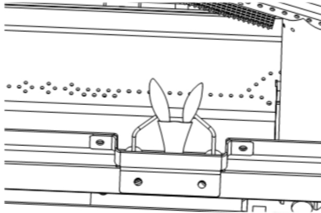
Figure 12.2 - Position correcte des flammes de veilleuse
