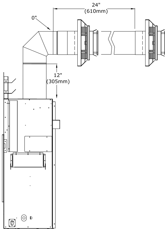
Figure 7.6 - Conduit 5 po x 8 po à terminaison horizontale
