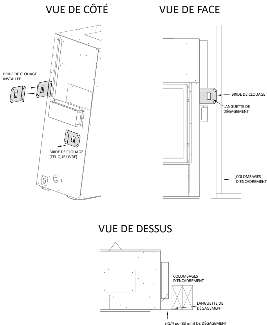
Figure 3.3 - Installation des brides de clouage
