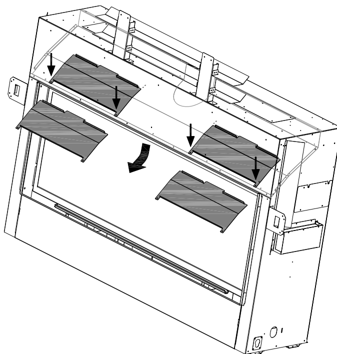
Figure 4.3 - Retrait des déflecteurs de convection
