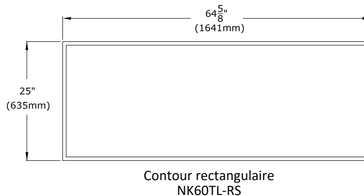
Figure 2.4 - Dimensions du contour (en option)
