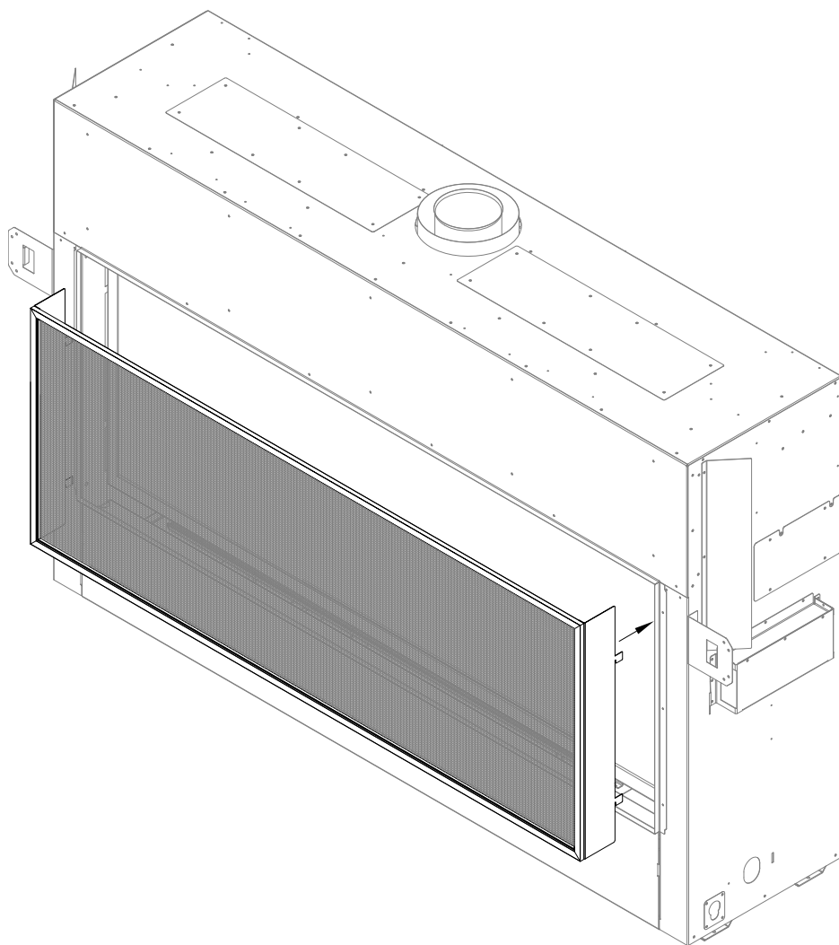
Figure 8.6 - Installation de l'écran pare-étincelles
