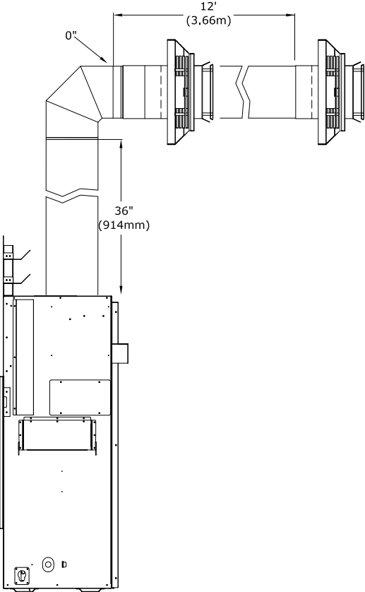
Figure 7.7 - Conduit 5 po x 8 po à terminaison horizontale
