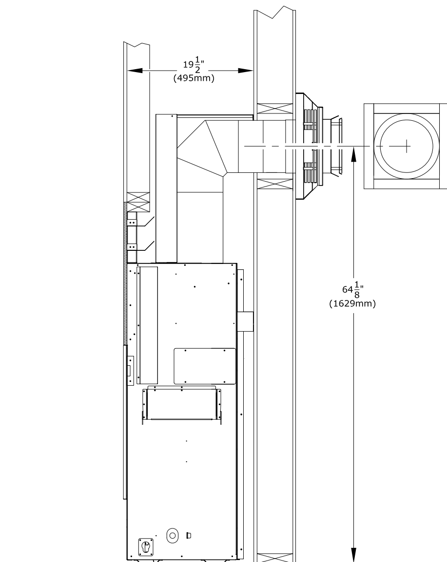
Figure 3.8 - Encadrement du coupe-feu mural (dimensions minimums)
