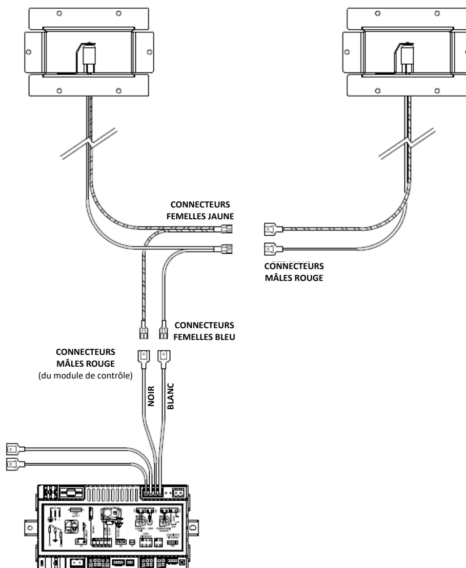
Figure 8.14 - Câblage du kit d'éclairage plafonnier
