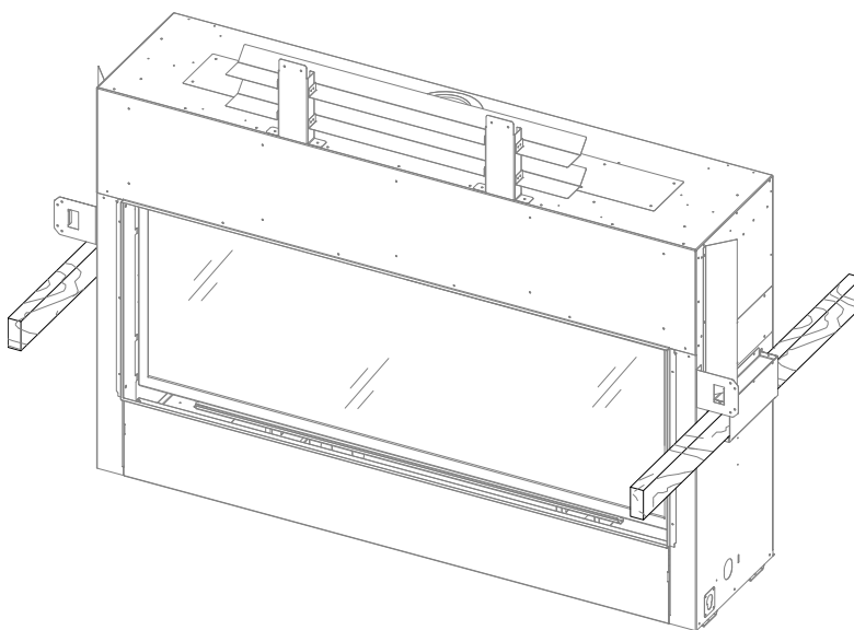
Figure 3.1 - Poignées de levage pour colombages 2"x4"
