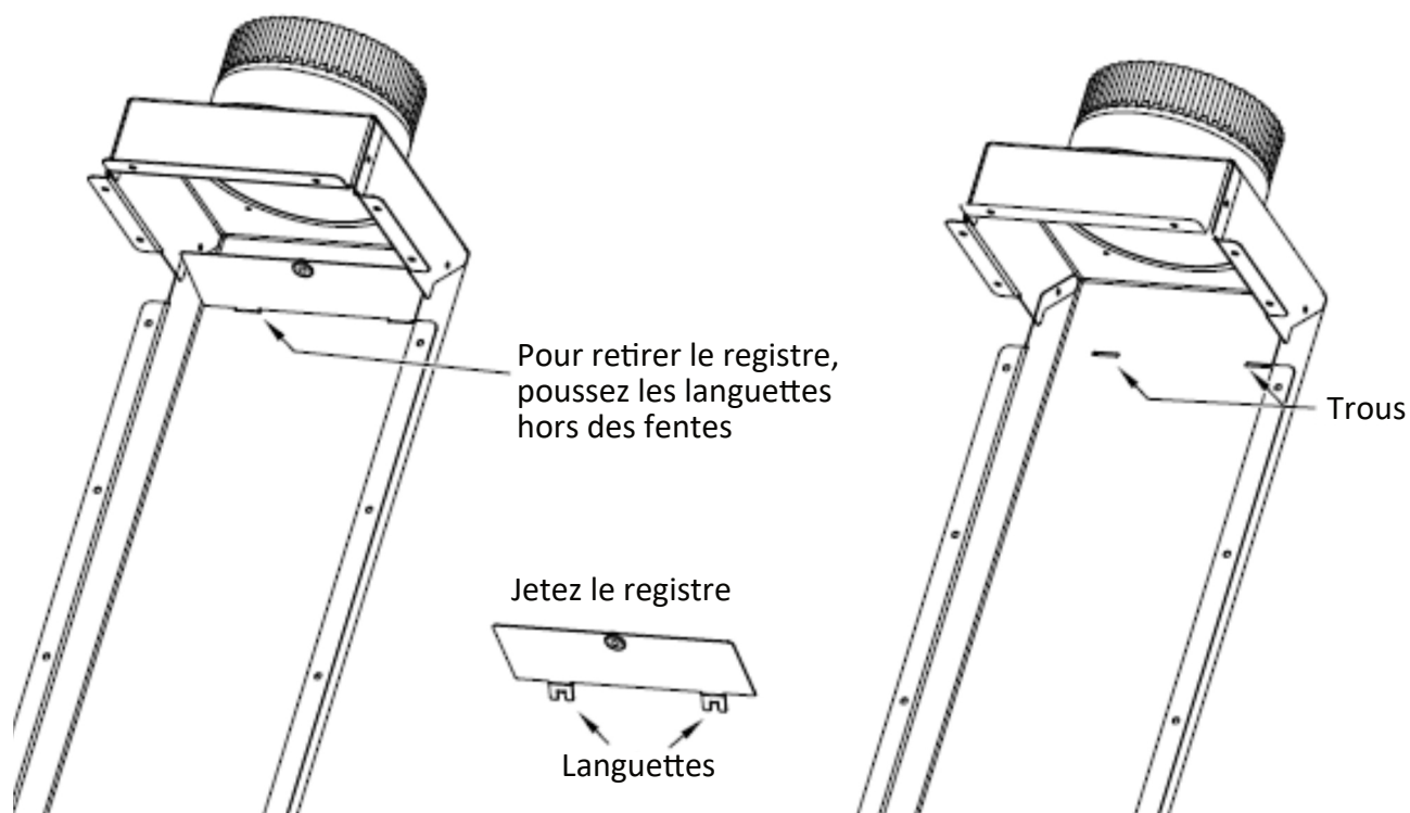
Figure 4.6 - Retrait du registre de chute d'air pour installer le kit HTK-INT
