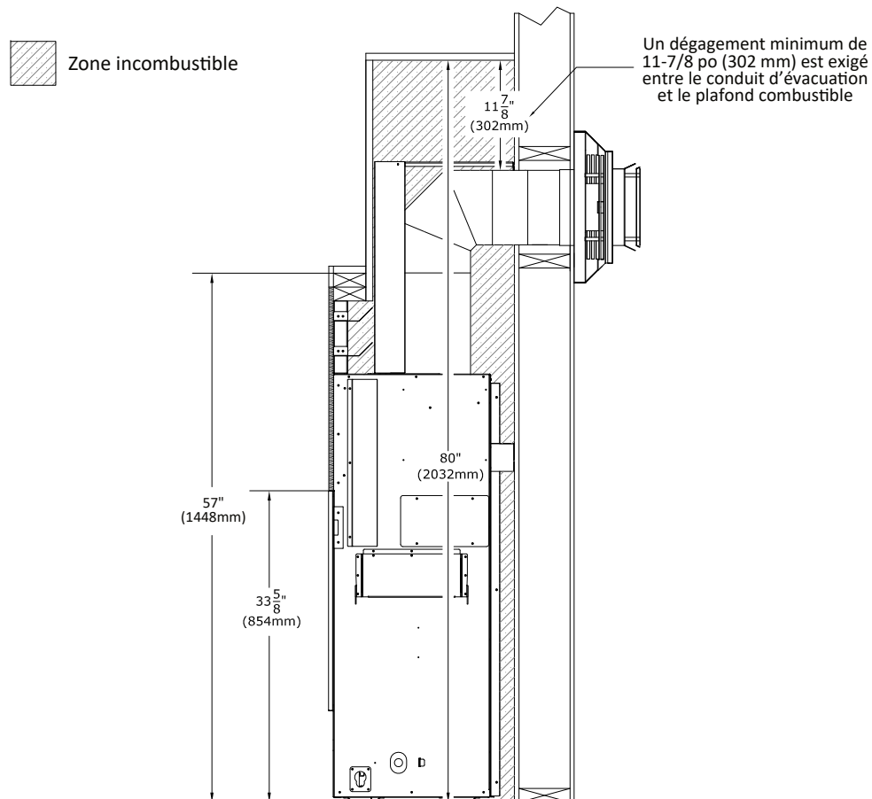
Figure 3.6 - Dégagements du conduit d'évacuation horizontal
