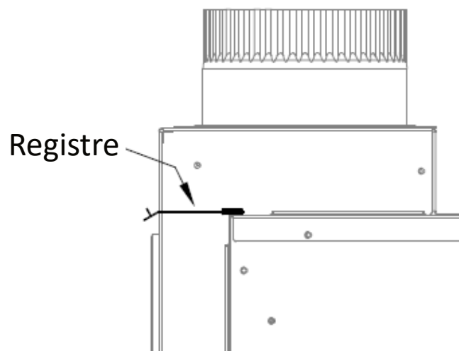
Figure 4.5 - Position de repos du registre de chute d'air (du kit HTK)
