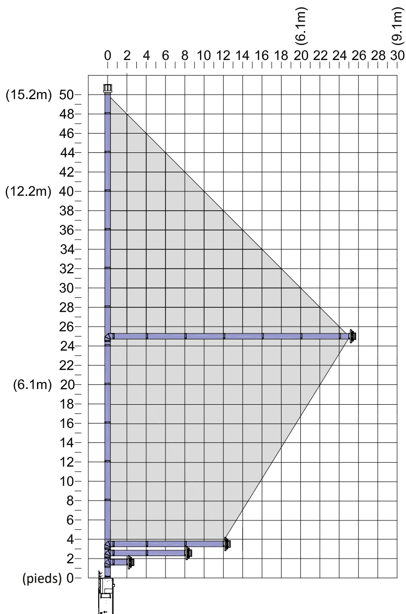
Figure 7.8 - Diagramme d'évacuation pour conduits combinés (V/H)
