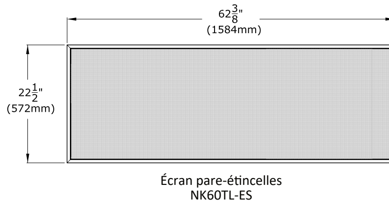
Figure 2.3 - Dimensions de l'écran pare-étincelles
