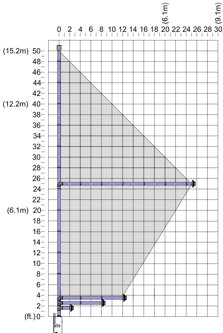
Figure 8.8 - Diagramme d'évacuation pour conduits 5 po x 8 po combinés (V/H)
