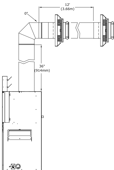
Figure 8.6 - Conduit 5 po x 8 po à terminaison horizontale
