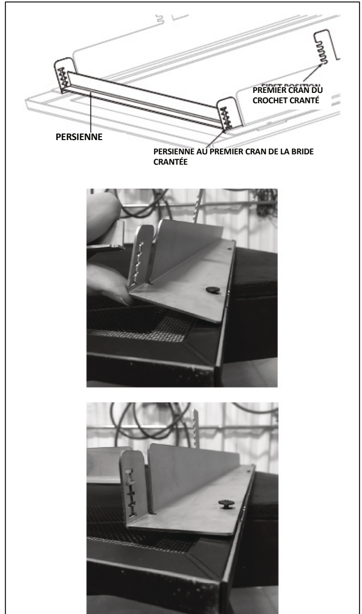
Figure 5.7 - Position de la persienne
