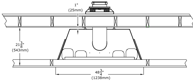
INSTALLATION TYPIQUE AVEC TERMINAISON HORIZONTALE
