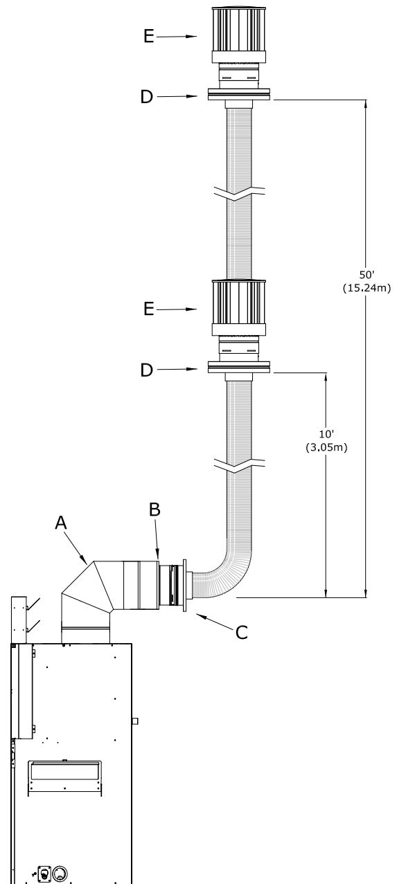
Figure 8.9 - Conversion de cheminée (Classe A/maçonnerie)
