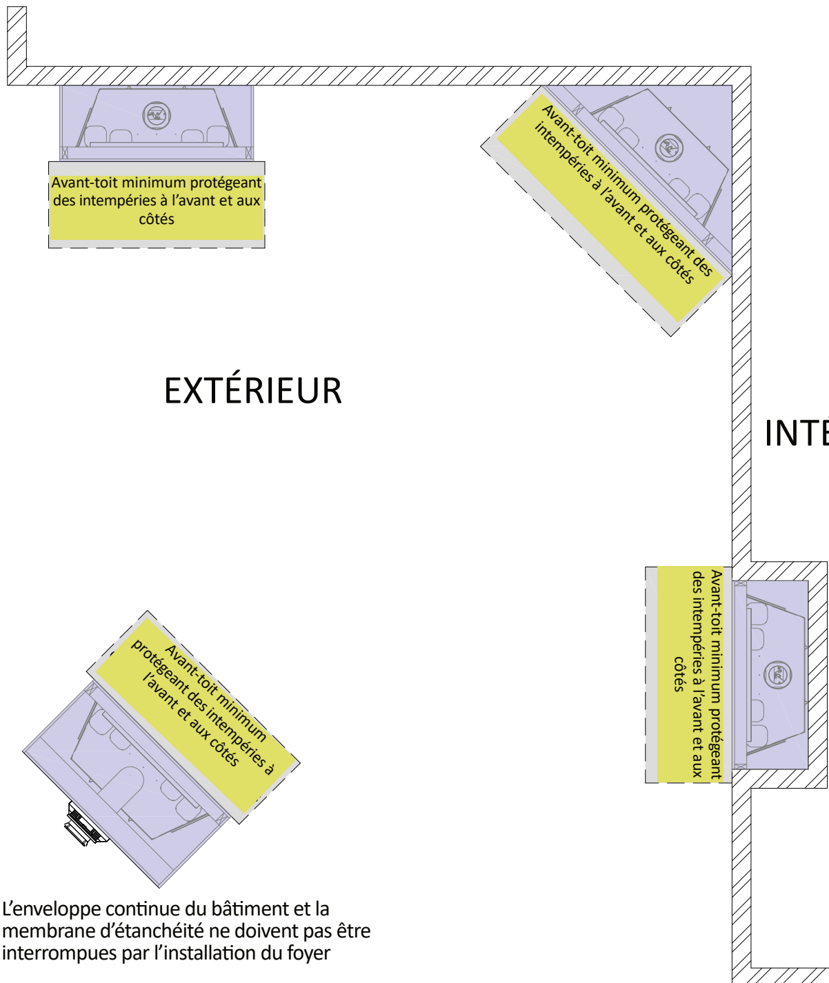
Figure 3.8 - Installation du foyer extérieur couvert
