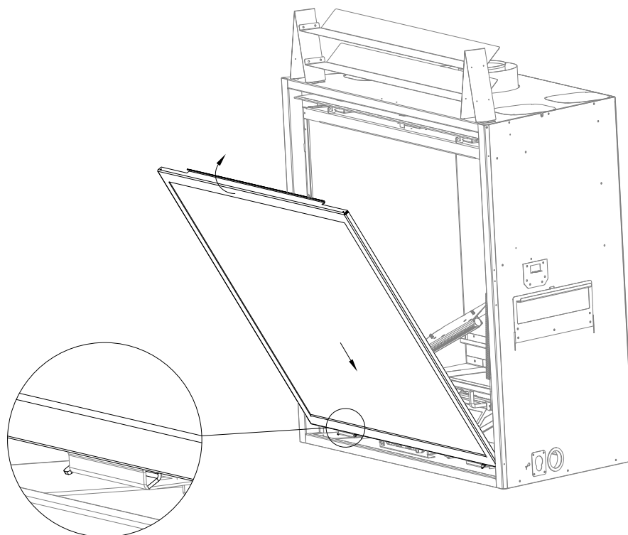
Figure 9.1 - Installation du cadre vitré
