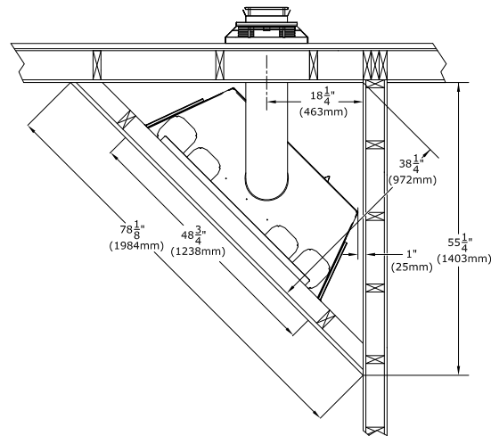
INSTALLATION TYPIQUE DANS UN COIN
