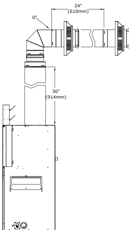
Figure 8.7 - Installation dans un sous-sol: Conduit 4 po x 6-5/8 po à terminaison horizontale
