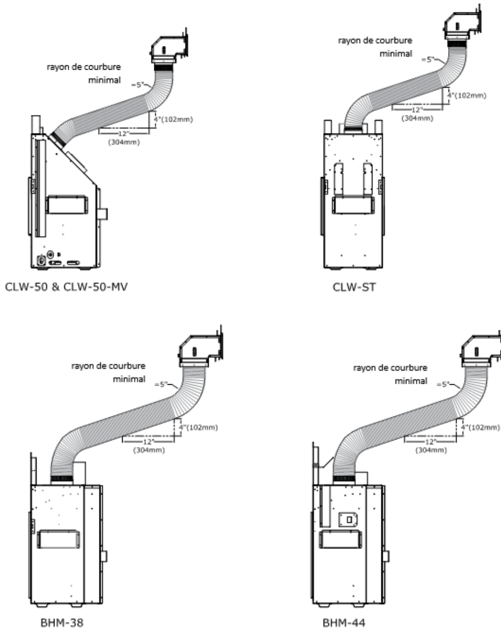
Figure 1.8 - Longueurs minimales du tuyau d'évacuation - seulement (1) plénum illustré
