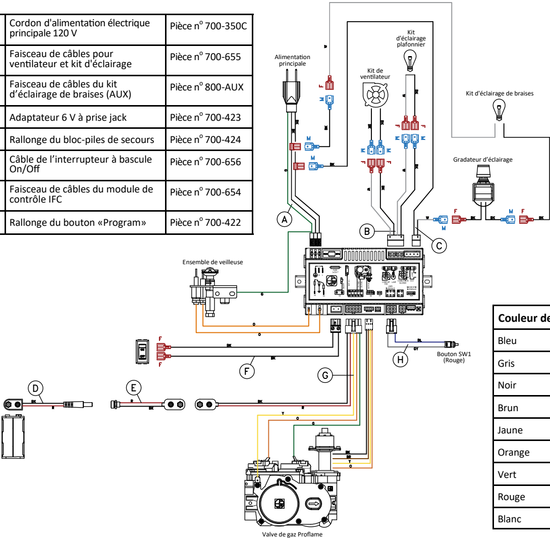
Figure 10.1 - Schéma de câblage
