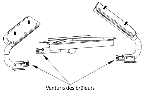
Figure 12.2 - Venturis des brûleurs
