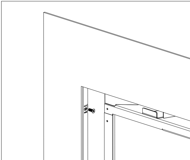
Figure 9.9 - Brides et écrous de fixation alignés
