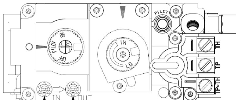
A) Robinet de pression d'entrée B) Prise de pression du collecteur
