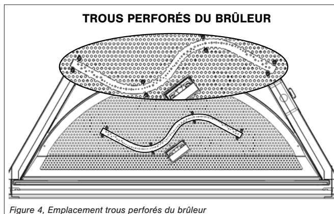
Figure 4, Emplacement trous perforés du brûleur
