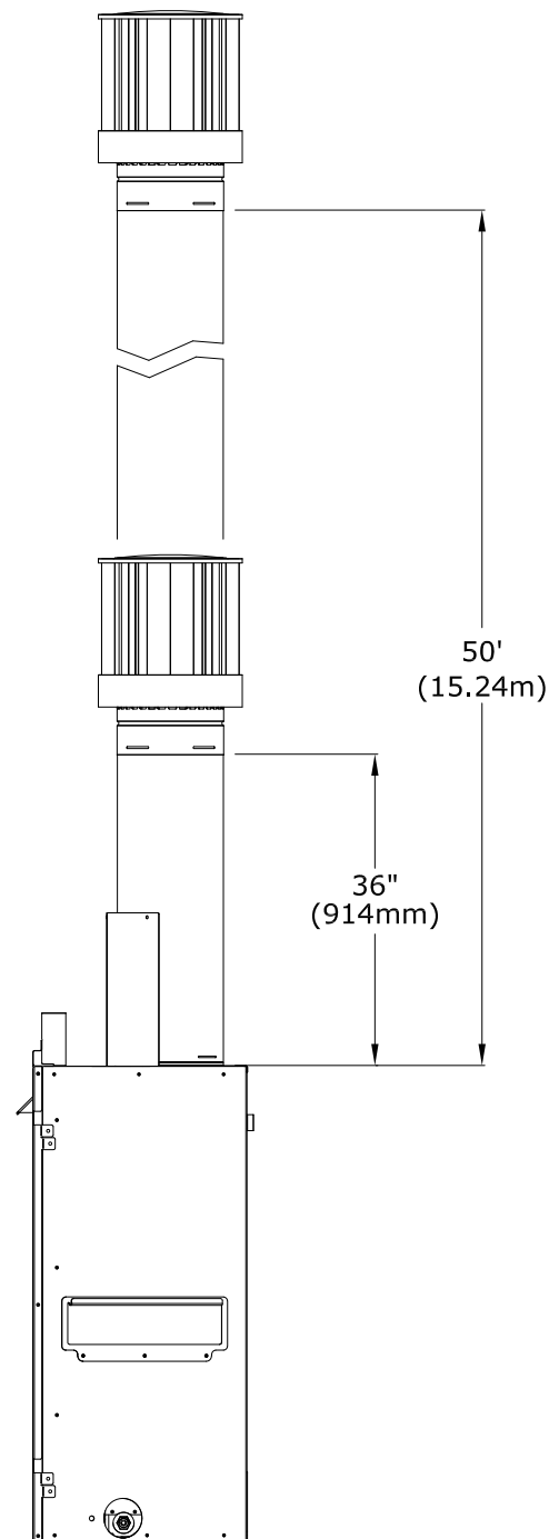
Figure 7.2 - Conduit 4"x6-5/8" à terminaison verticale
