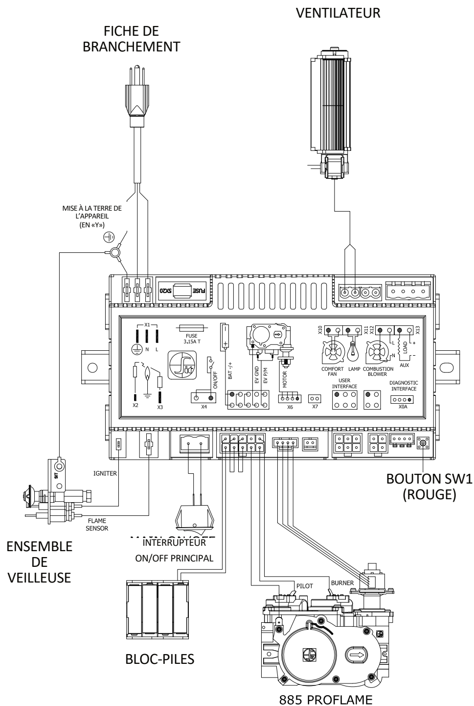
Figure 9.1 - Schéma électrique du SP-41-L
