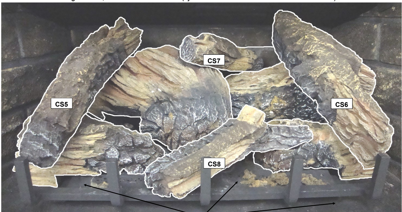
Figure 8.6b, Jeu de bûches installé (ajout des clinkers et braises en laine de roche)
